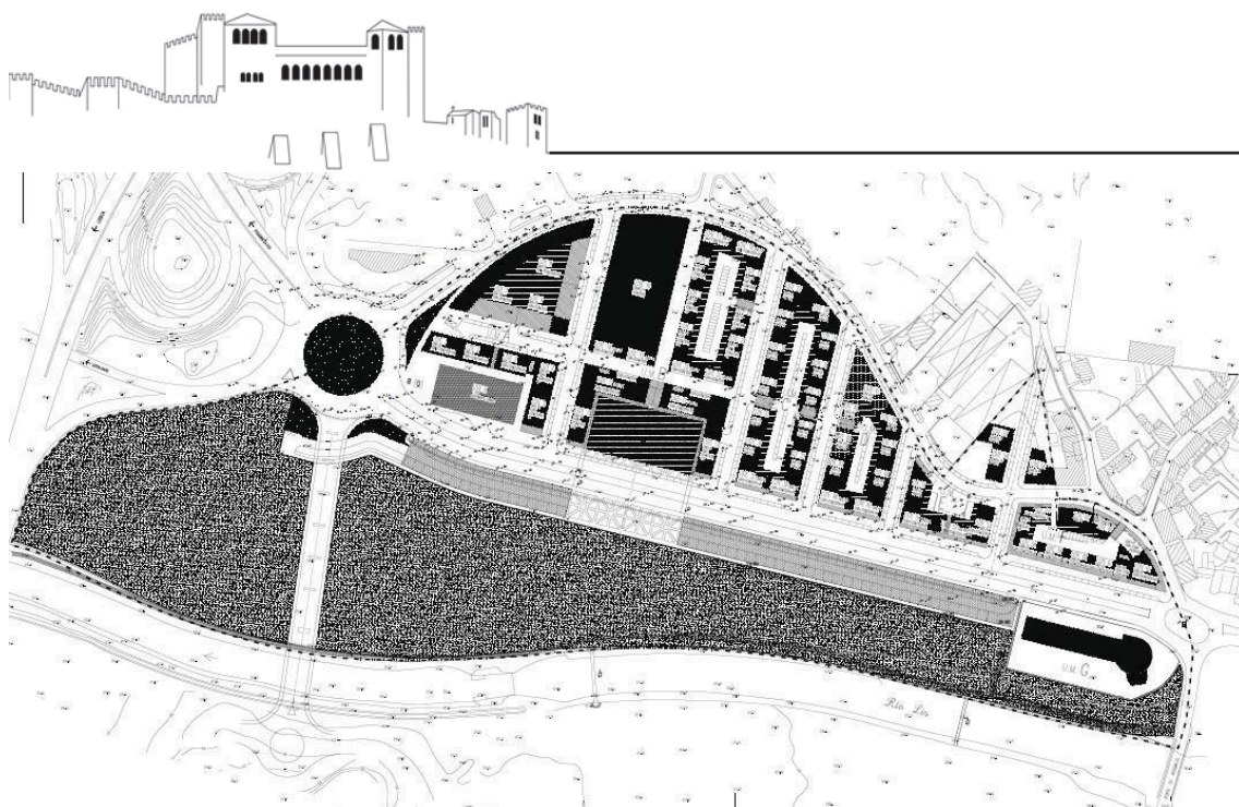
Fig.9 – Planta do PP da Almuinha com a alteração apresentada em Conferência de Serviços em 2 de dezembro de 2013.
