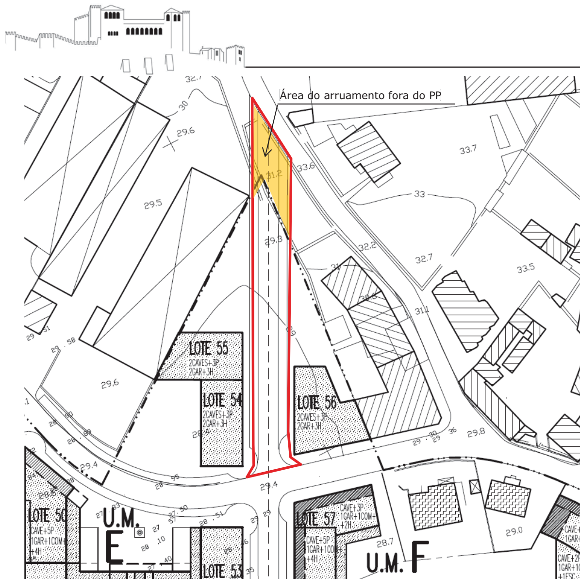
Fig.12 – Planta do troço do arruamento "E" que falta executar.
