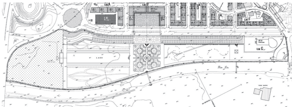
Fig. 4 – Planta do PP da Almoinha conforme publicado na página 3874 do DR I série B n.º 92 de 19-04-2002
