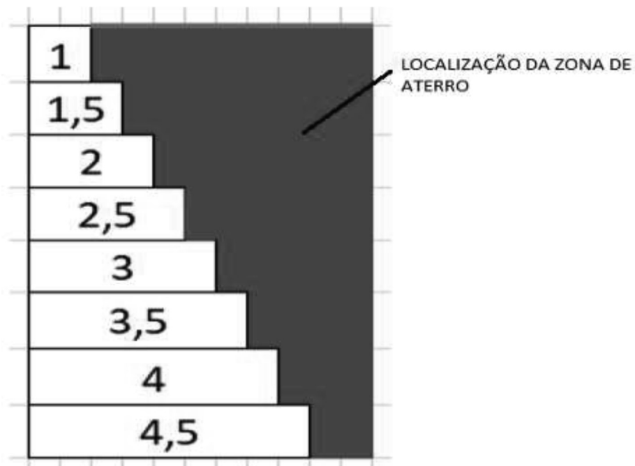
Fig. 4 - Corte esquemático do Muro de Gabiões
