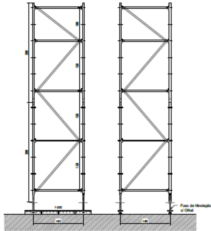
Alçados Esc:1/50
