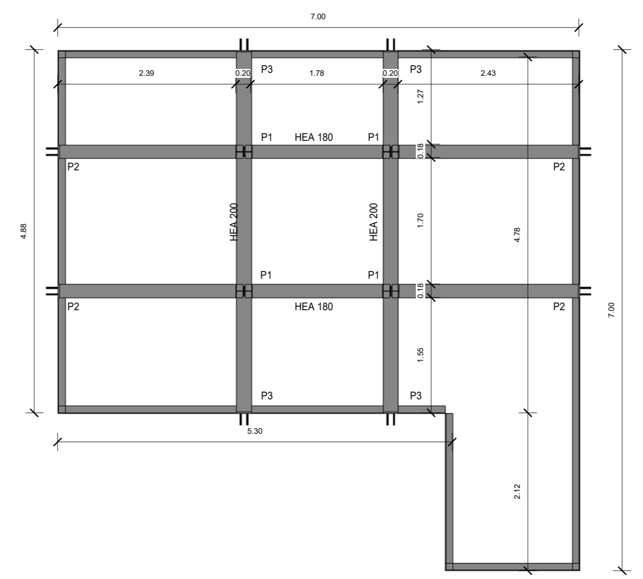
SOLUÇÃO DE REFORÇO DA LAJE 79 1:50
