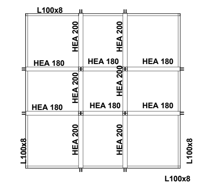
Modulo de Reforço Lajes (ver Porm em EST.02)
