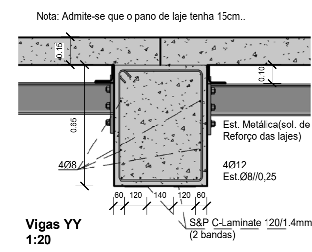
Vigas YY 1:20
