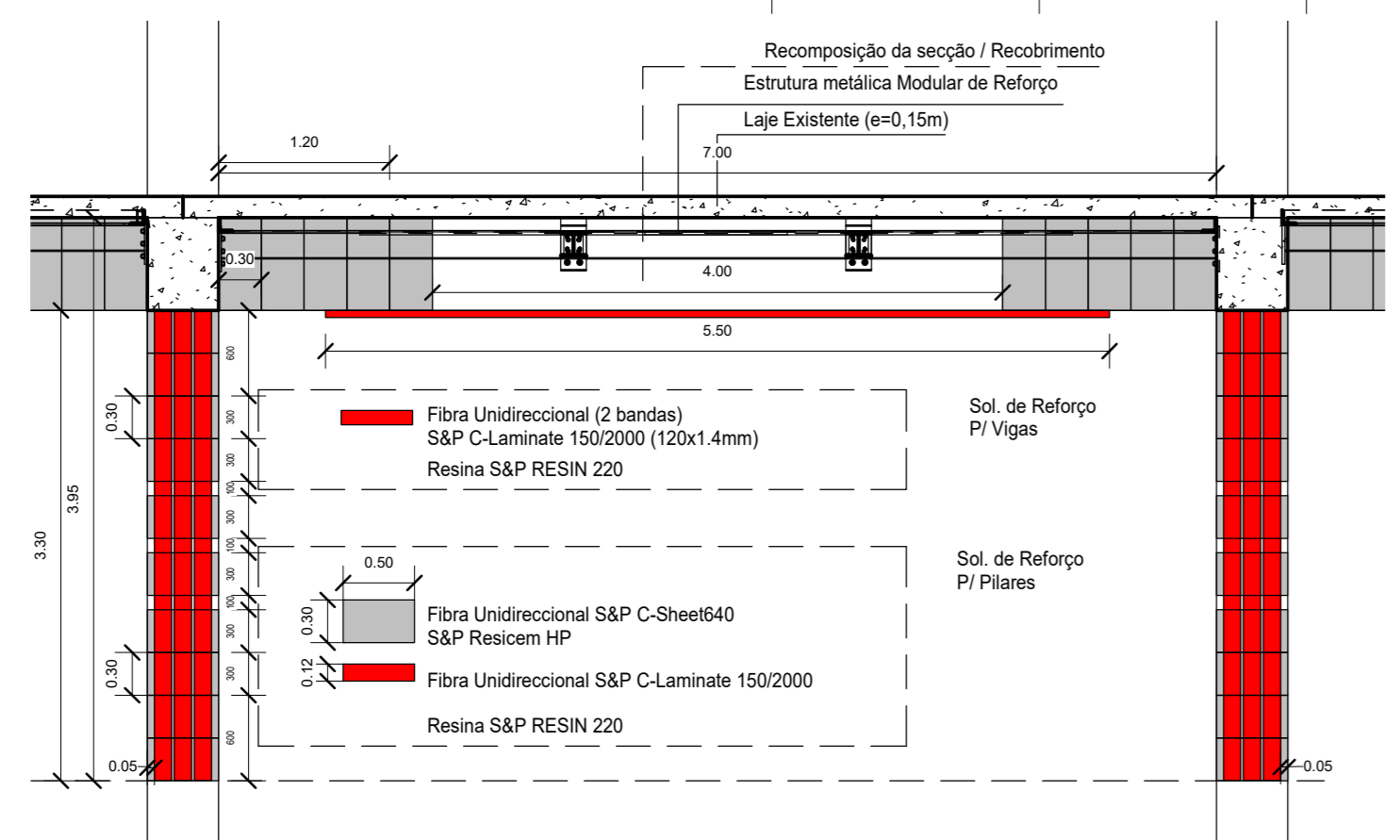
Modulo de Reforço Lajes (ver Porm em EST.02)
