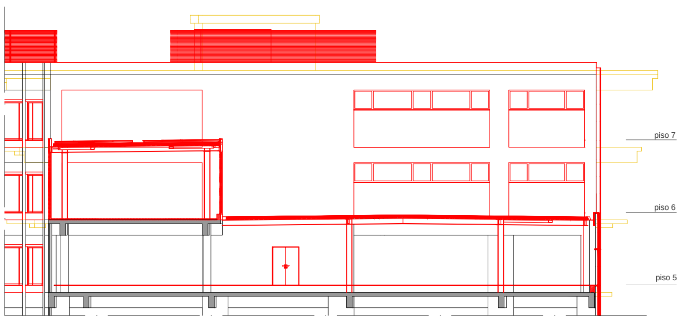
ALÇADO NASCENTE (TORRE POENTE)
