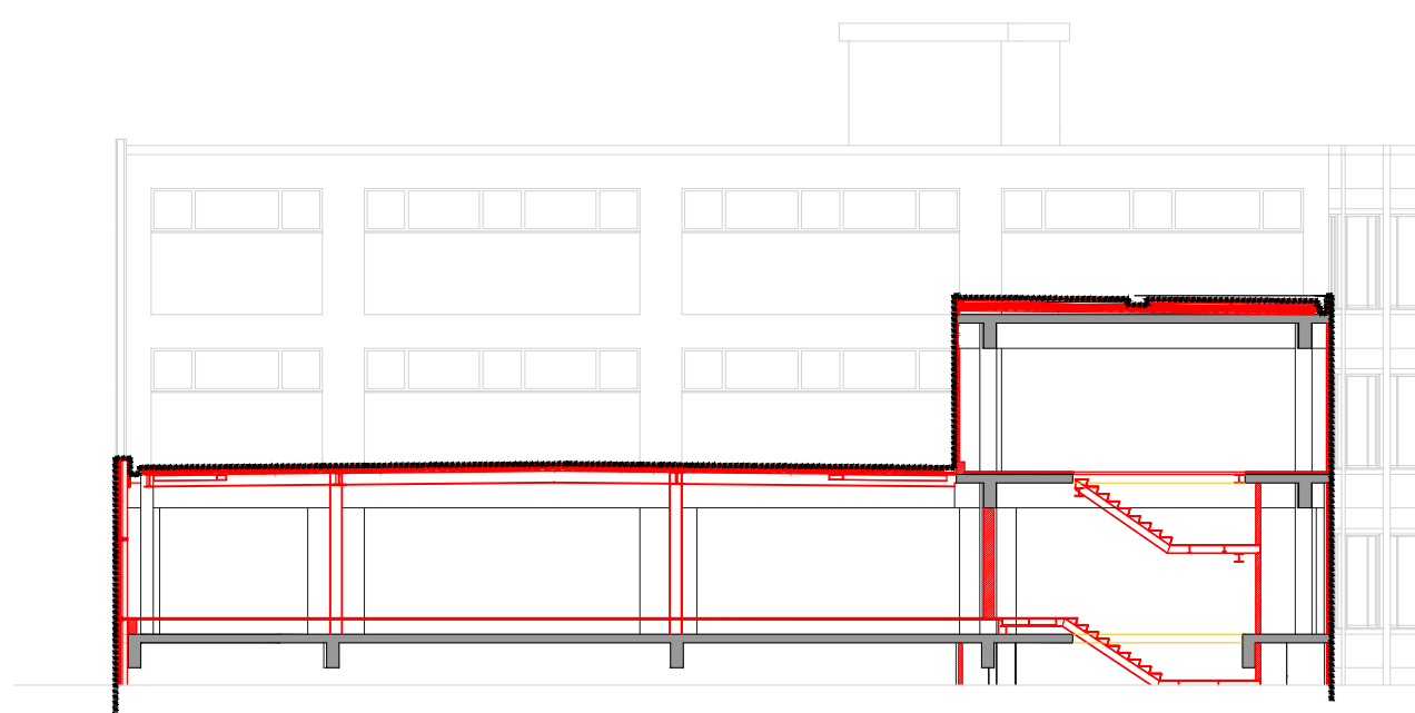
ALÇADO POENTE (TORRE NASCENTE)
