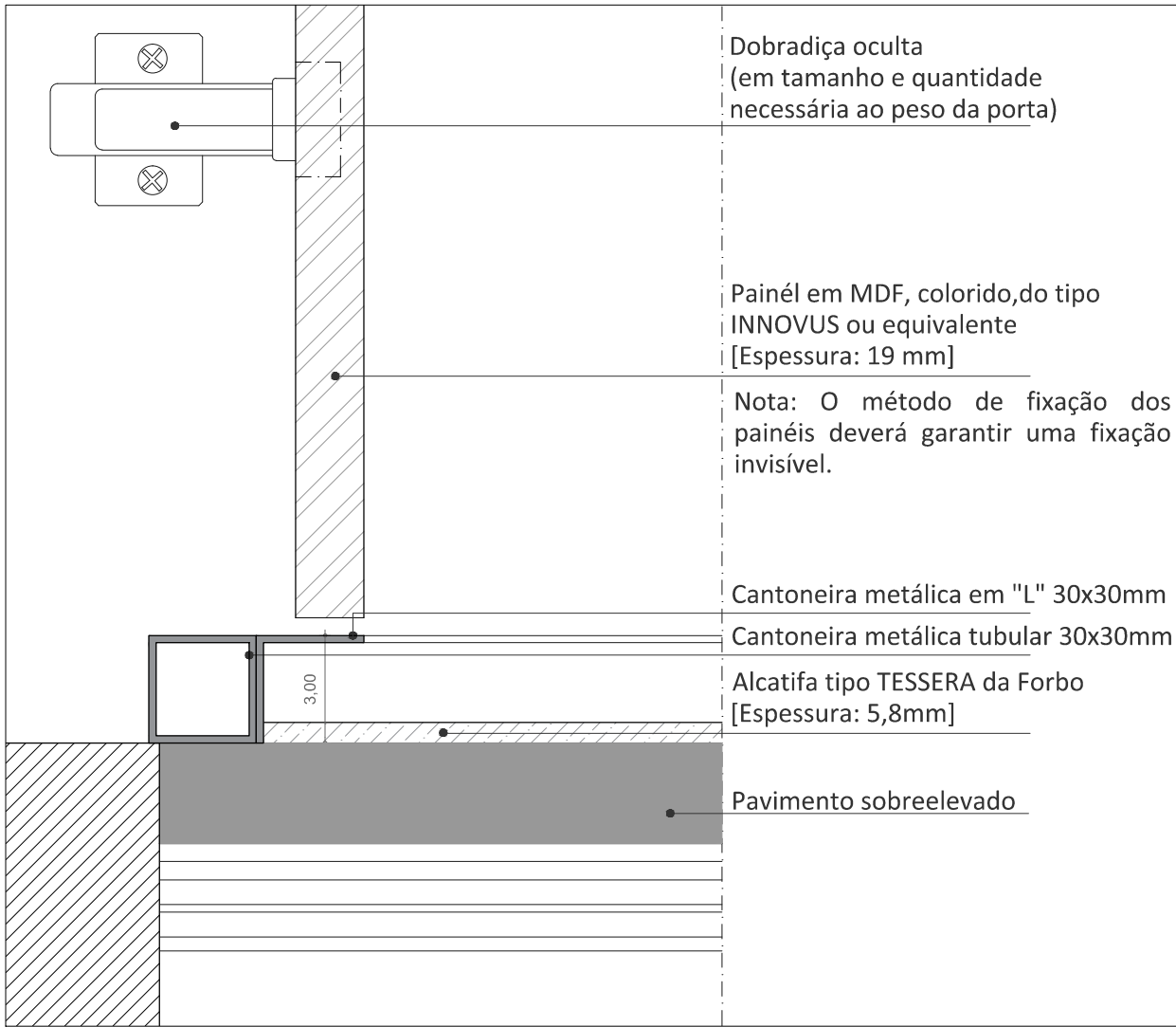
P2 - PORMENOR INTERSEÇÃO DE PORTA COM ACABAMENTO MDF E PAVIMENTO - 1:2
