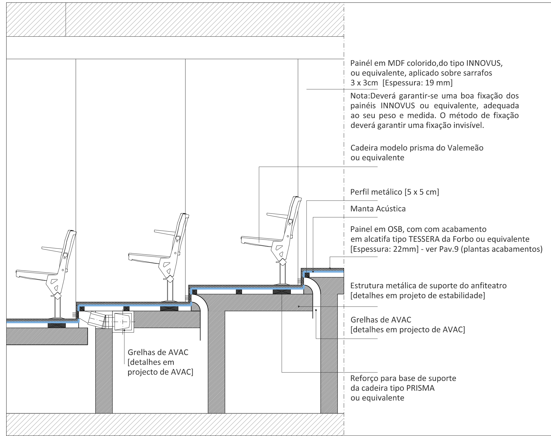
P1 - CORTE BANCADAS - ESTRUTURA E GRELHAS DE VENTILAÇÃO 1:20
