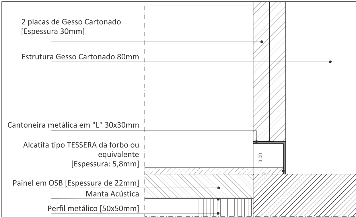
P4 - PORMENOR INTERSEÇÃO DE PAREDE GESSO CARTONADO E PAVIMENTO - 1:2
