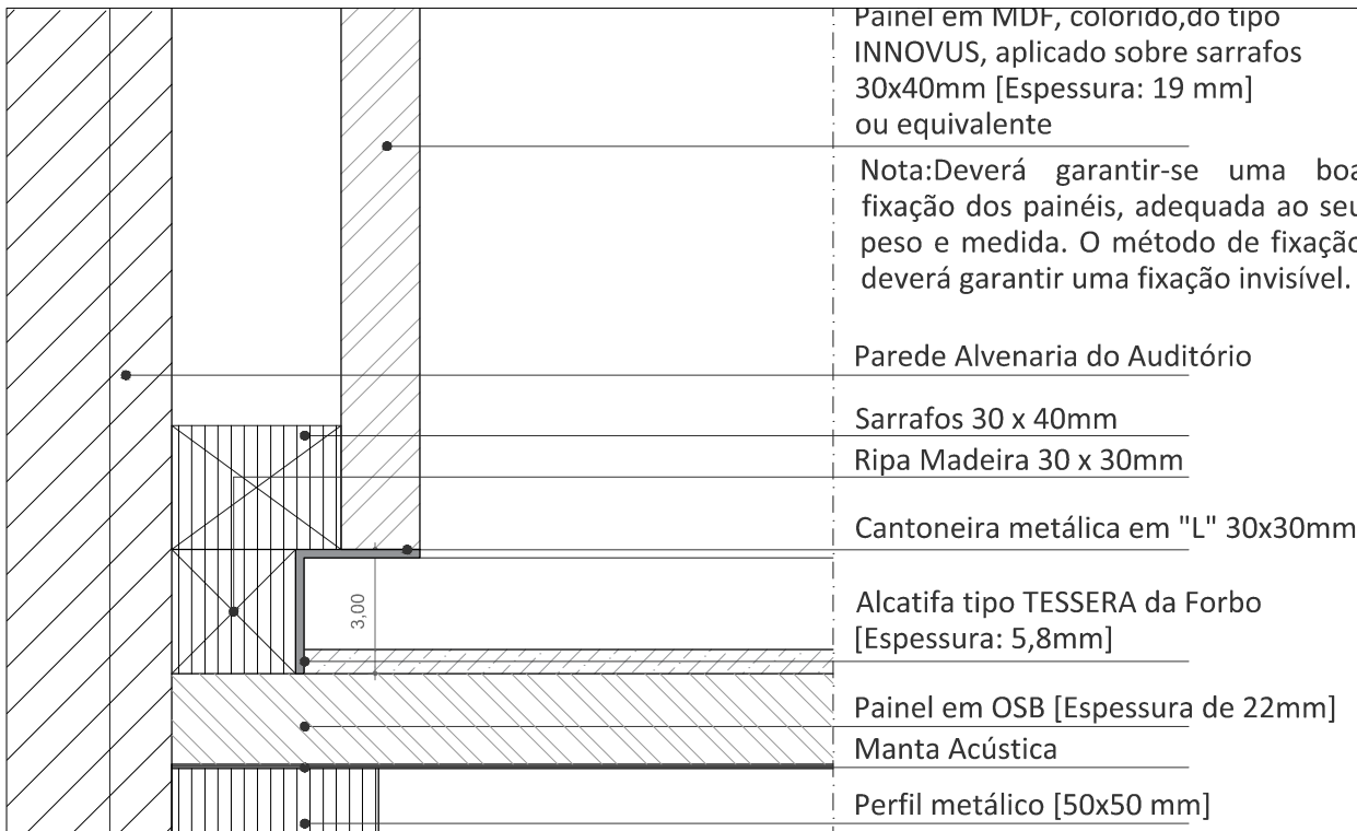
P3 - PORMENOR INTERSEÇÃO DE PAREDE ALVENARIA COM ACABAMENTO EM MDF E PAVIMENTO - 1:2
