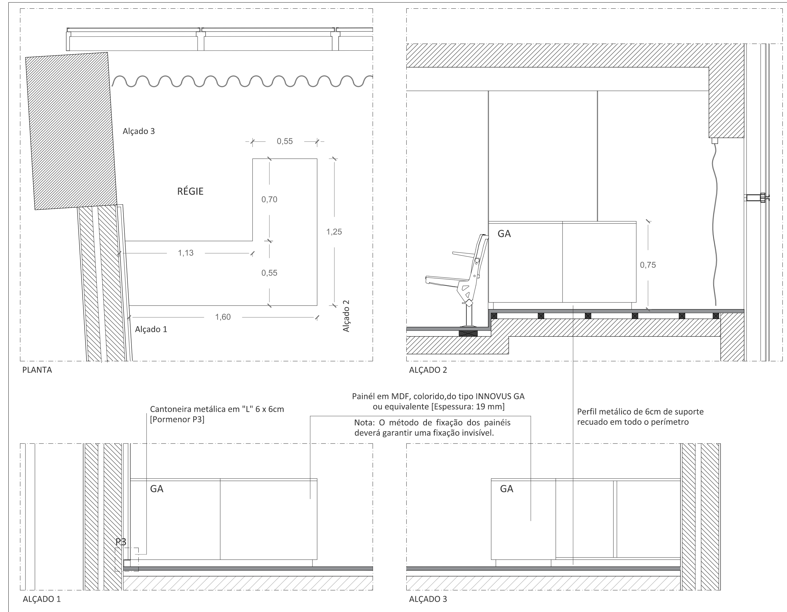
RÉGIE - PLANTA E ALÇADOS 1:20
