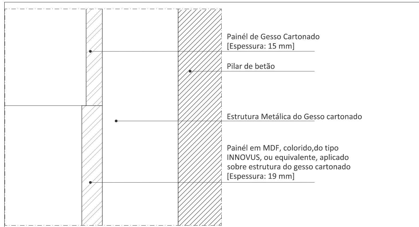
P1 - CORTE VERTICAL PELA JUNÇÃO DO ACABAMENTO EM MDF E GESSO CATONADO - 1:2
