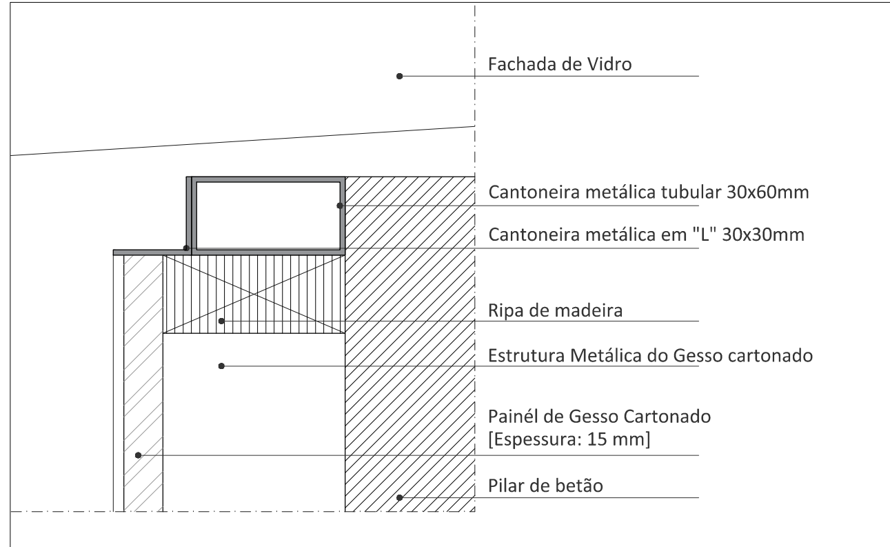
P3 - CORTE HORIZONTAL NA JUNÇÃO DO ACABAMENTO EM GESSO CARTONADO COM FACHADA DE VIDRO
