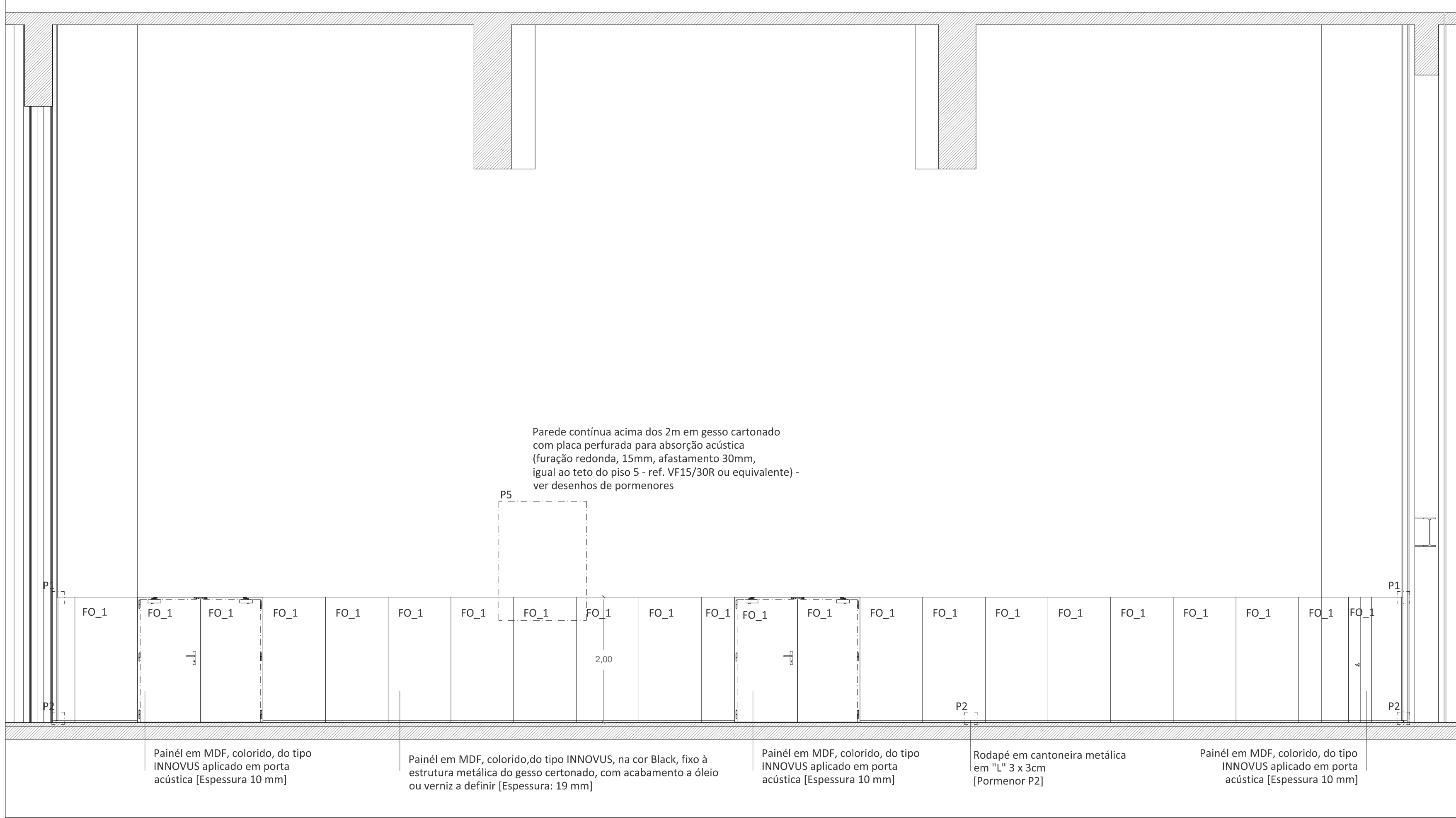
CORTE BB'
