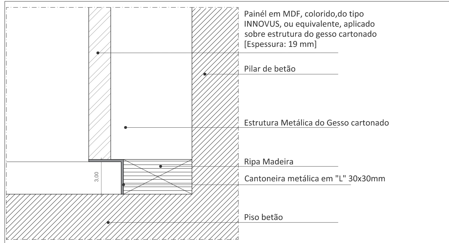
P2 - CORTE VERTICAL PELA JUNÇÃO DO ACABAMENTO EM MDF E PAVIMENTO - 1:2
