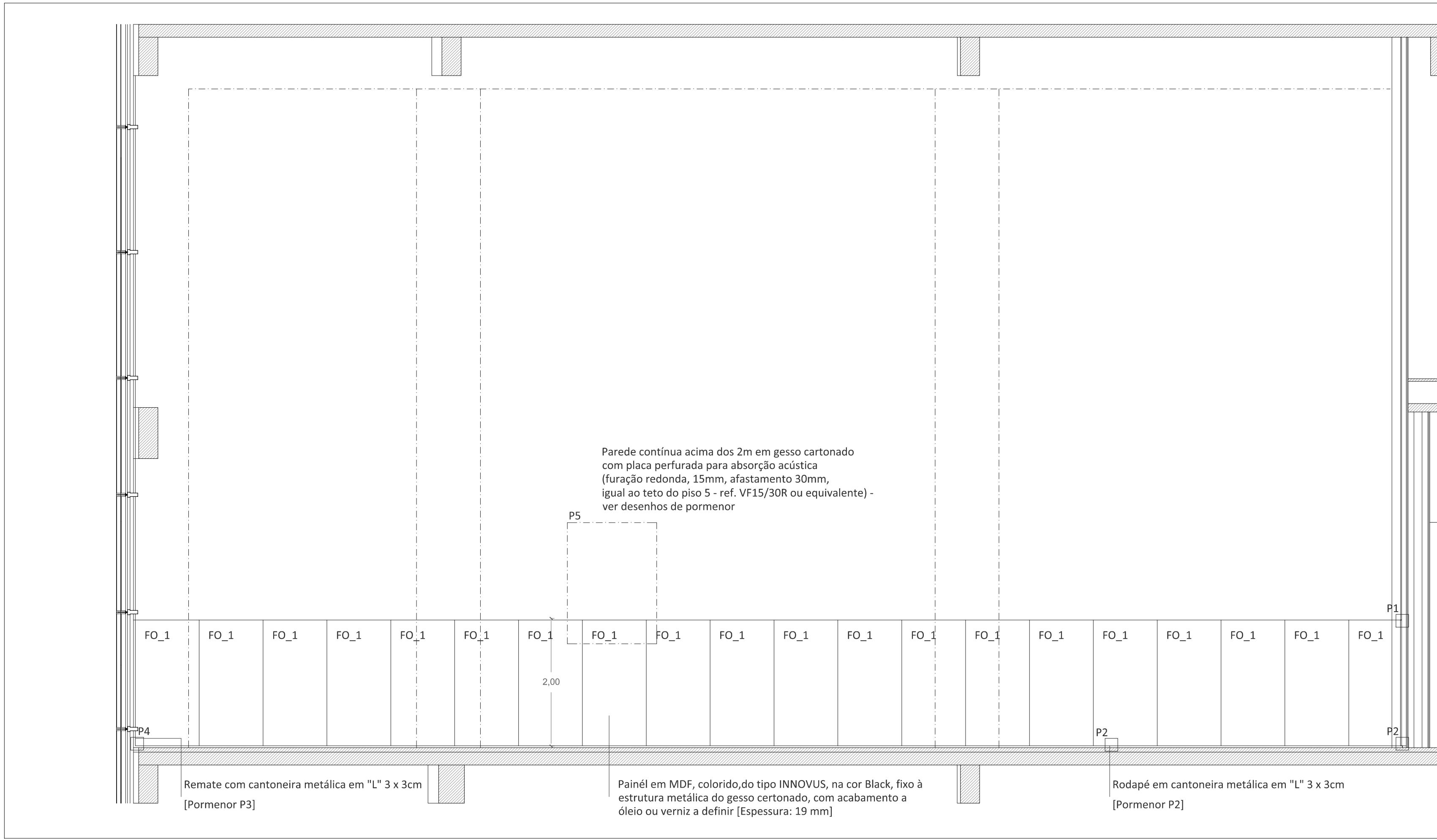
CORTE CC'
