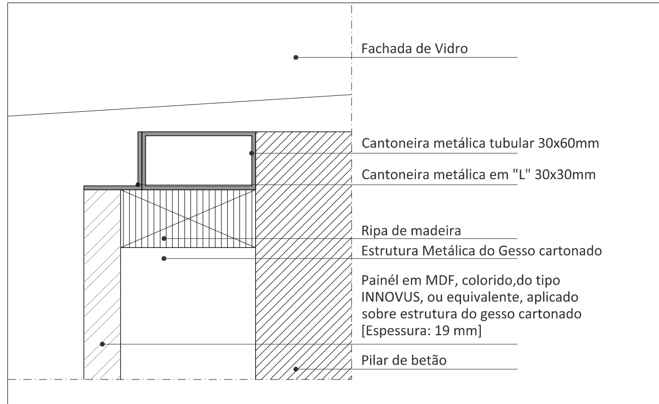
P4 - CORTE HORIZONTAL NA JUNÇÃO DO ACABAMENTO EM MDF COM FACHADA DE VIDRO
