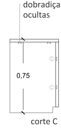
corte C
