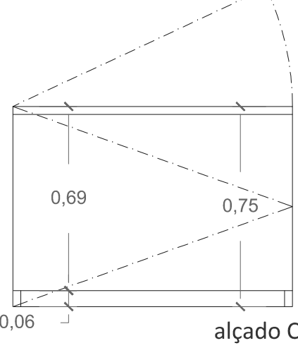
alçado C
