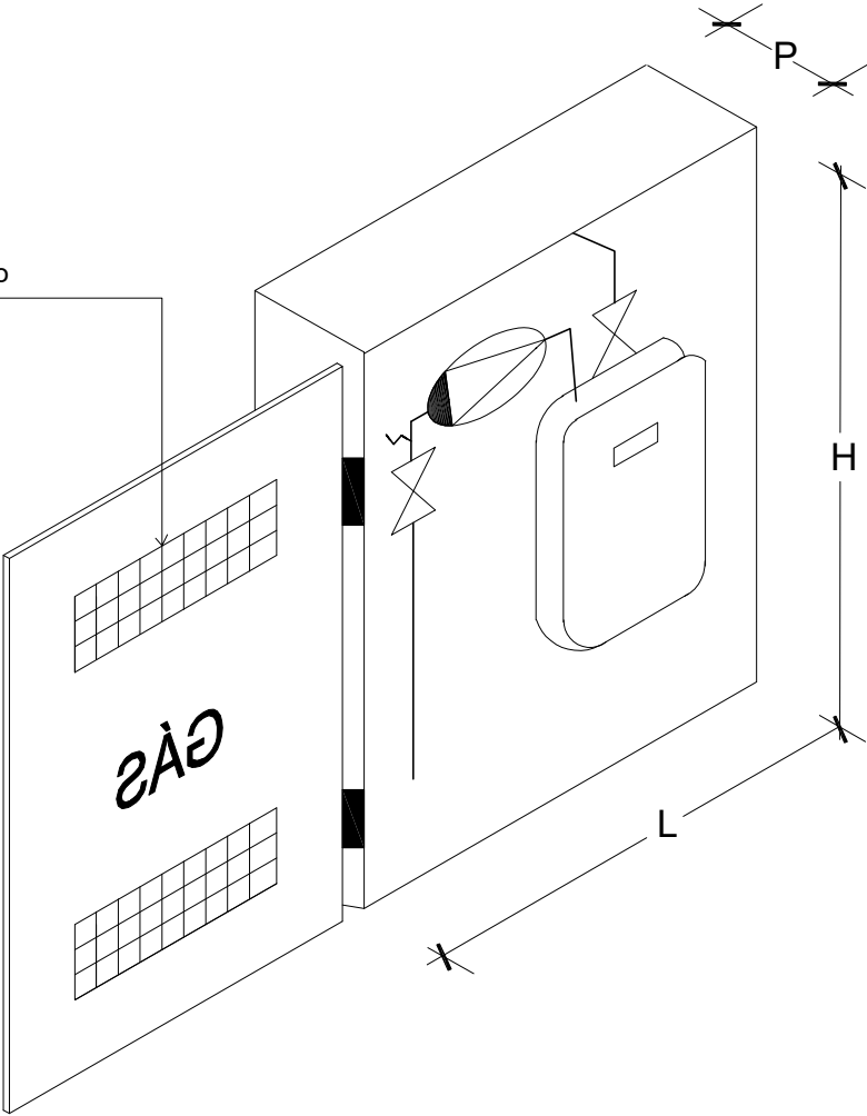
MEDIDAS DAS CAIXAS DOS CONTADORES
