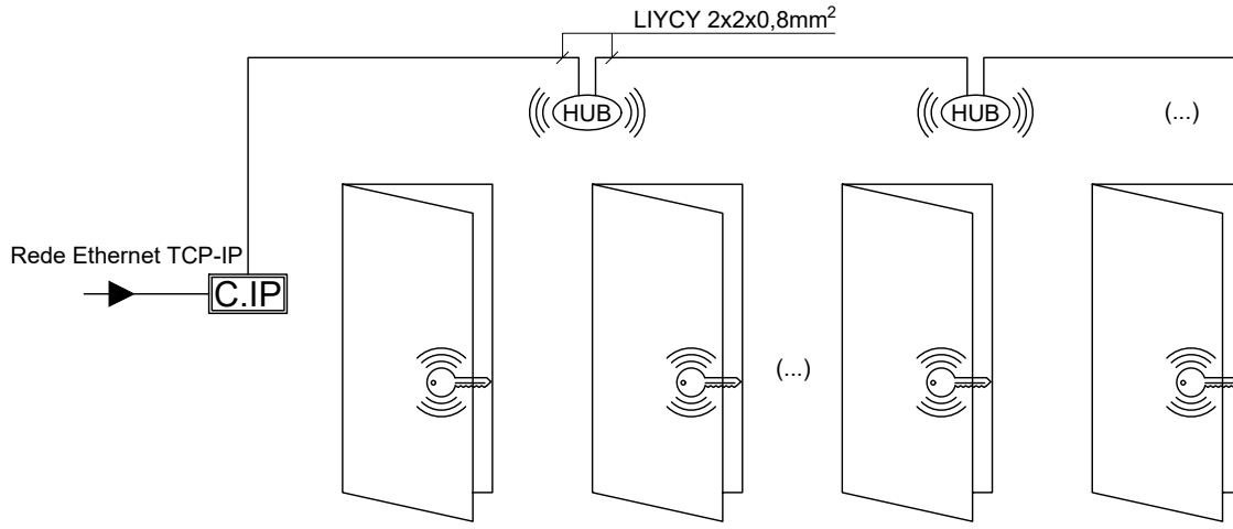
Diagrama Tipo Controlo de Acessos com Fechadura autónoma
