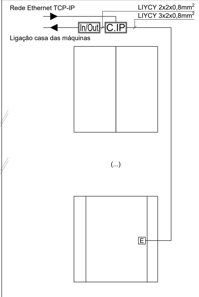
Diagrama Tipo Controlo de Acessos Elevador Panorâmico
