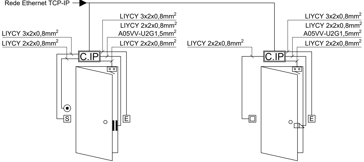
Diagrama Tipo Controlo de Acessos com Fechadura autónoma
