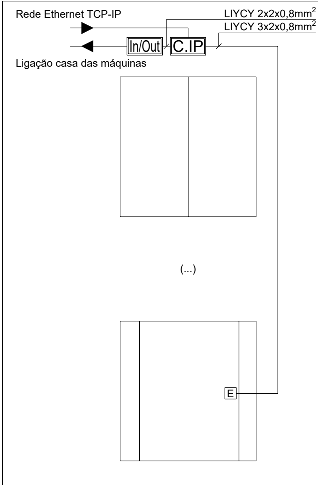
Diagrama Tipo Controlo de Acessos Elevador Panorâmico
