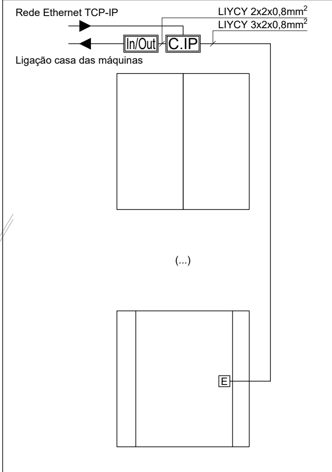
Diagrama Tipo Controlo de Acessos Elevador Panorâmico
