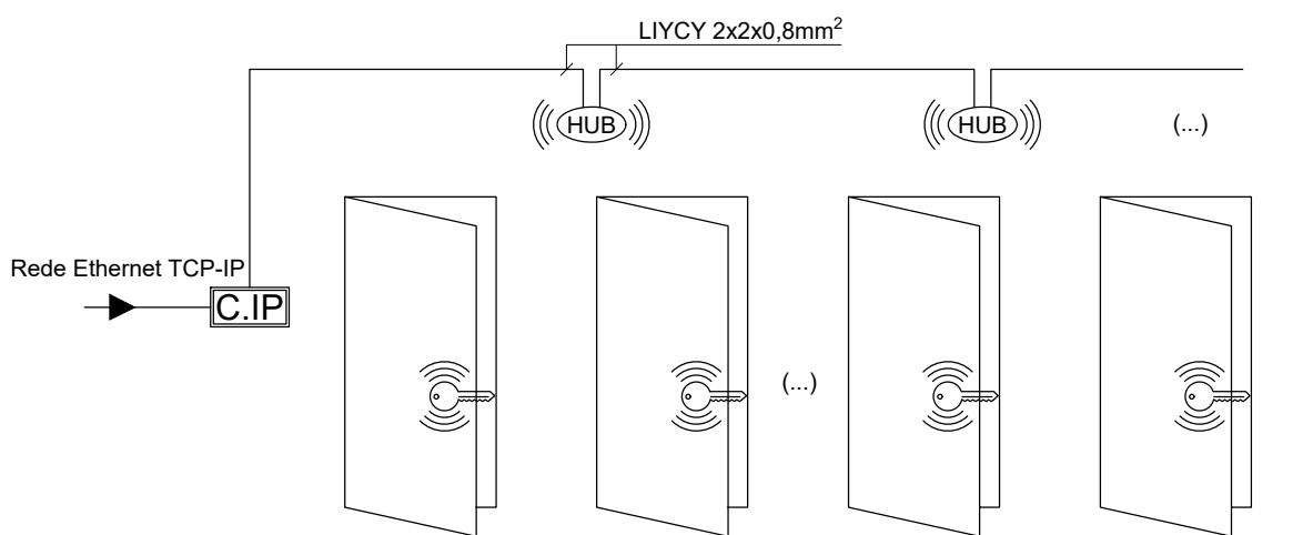
Diagrama Tipo Controlo de Acessos com Fechadura autónoma
