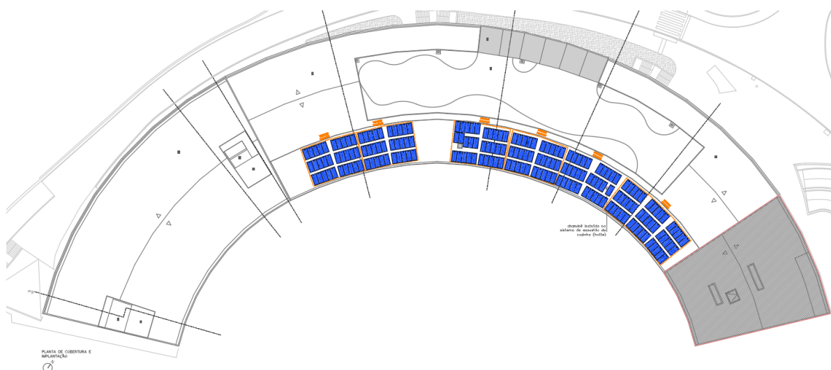
Figura 1 – Área de implantação para os painéis Fotovoltaico numa cobertura do Edifício.
