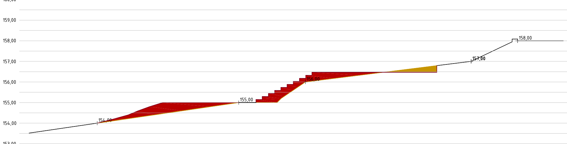
SECÇÃO / PERFIL DD
