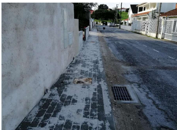
Figura 47 - execução de trabalhos relacionados com a execução de rede de drenagem pluvial e construção de passeios e bermas revestidas a pavê
