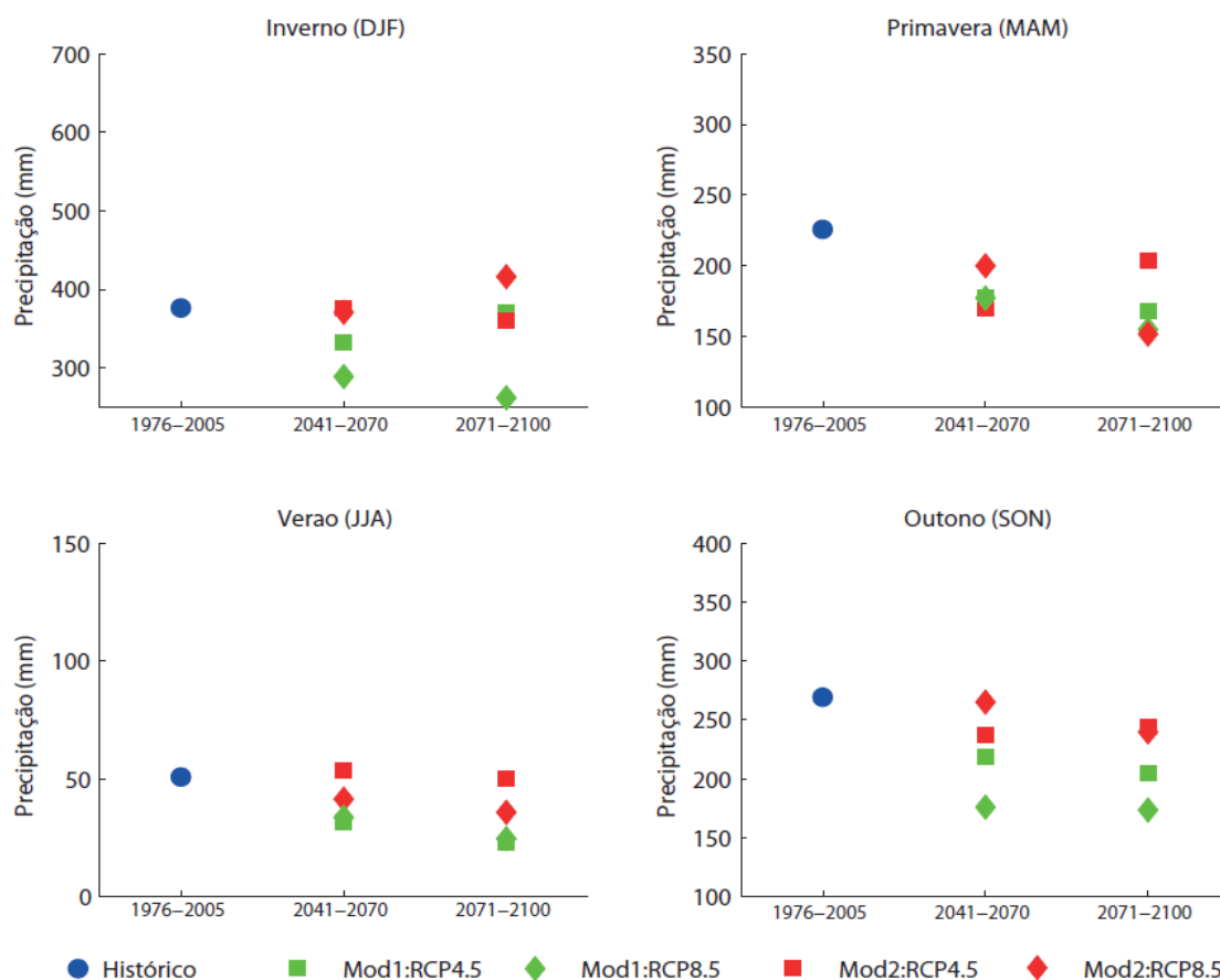
Figura 8 - Projeções da precipitação média (mm) por estação do ano (medias sazonais), para ambos os modelos e cenários, até ao final do século
