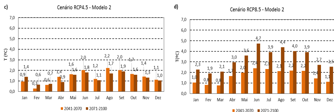
Figura 7 - Projeção das anomalias da média mensal da temperatura máxima (°C), para ambos os modelos e cenários, até ao final do século para o Município de Leiria
